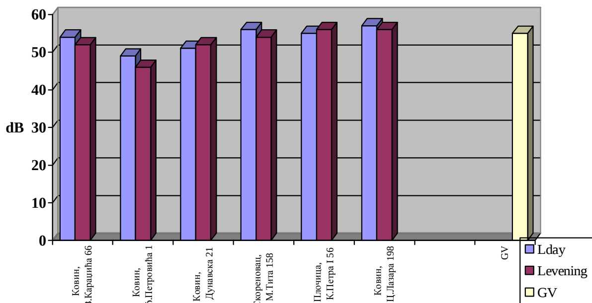
Графикон 15. Дневни и вечерњи ниво буке и гранична вредност индикатора буке за дан и вече у dB(A), на мерним местима у зони становања: Ковин, Скореновац, Плочица
