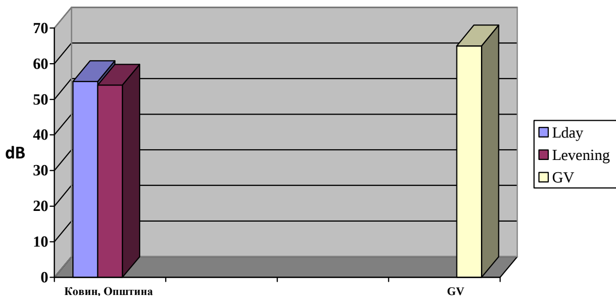
Графикон 1. Дневни и вечерњи ниво буке и гранична вредност индикатора буке за дан и вече у dB(A),радним даном, на мерном месту у зони градског центра: Ковин, Општина
