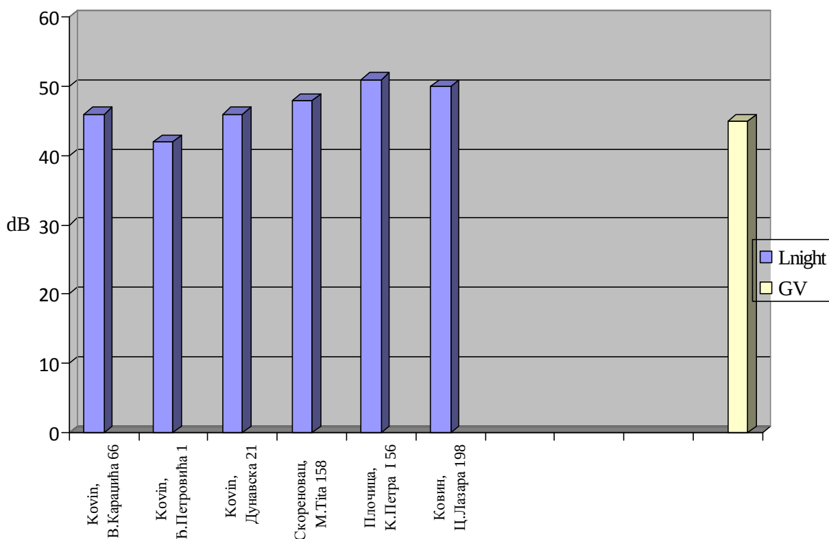
Графикон 16. Ноћни ниво буке и гранична вредност индикатора буке за ноћ у dB(A), на мерним местима у зони становања: Ковин, Скореновац, Плочица
