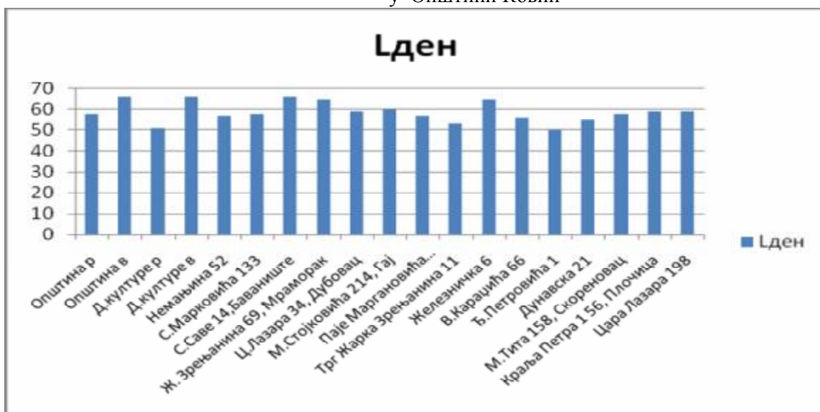
Графикон 18. Целодневни ниво буке у dB(A) на мерним местима у Општини Ковин
