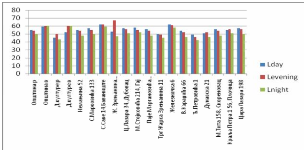
Графикон 17. Дневни, вечерњи и ноћни нивои буке у dB(A) на мерним местима у Општини Ковин
