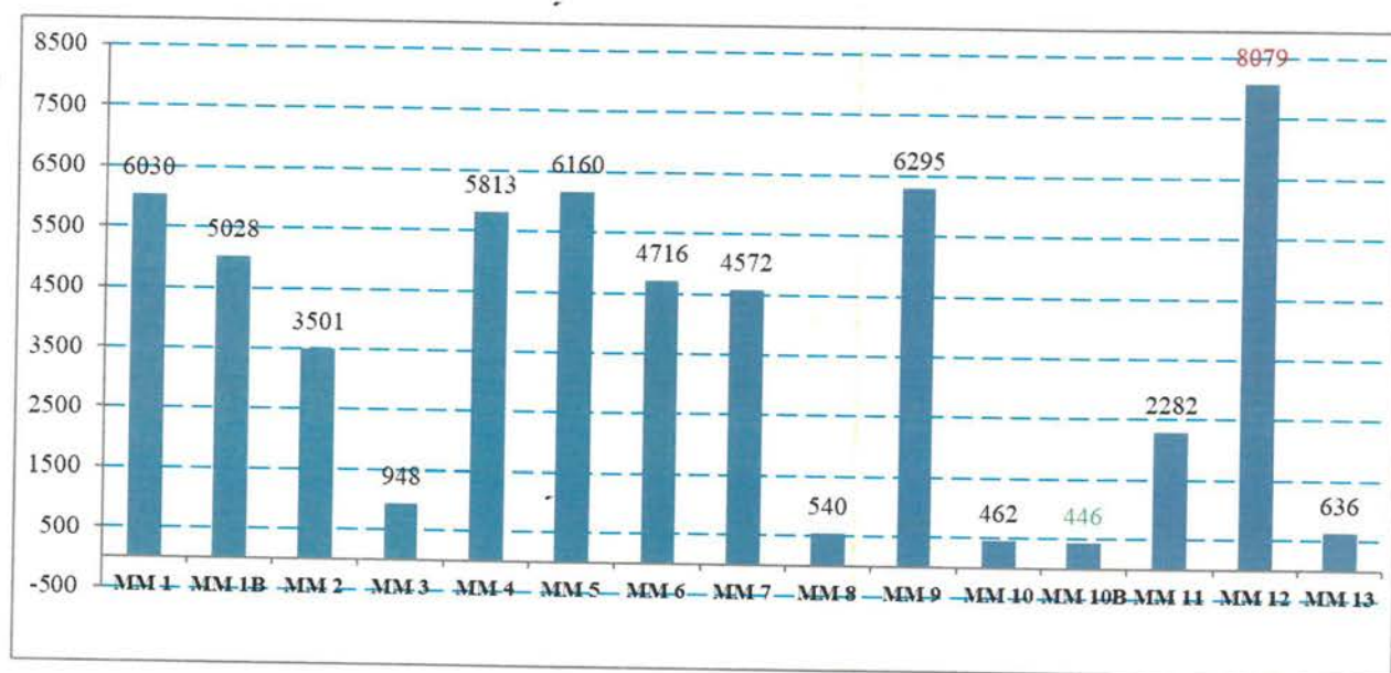
Графикон 1. Оптерећеност саобраћајем по мерним местима проласком лакхих возила
